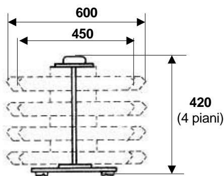
6580.396-397-398-399-400 KIT assemblaggio senza i contenitori
