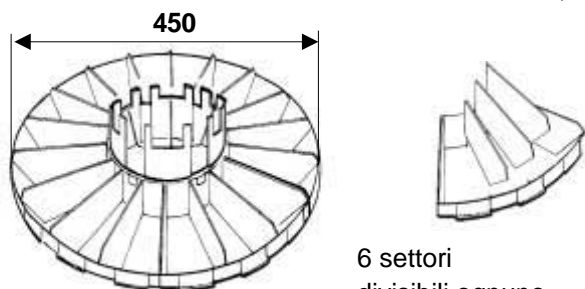
6580.390 arancio 6580.391 ESD nero
